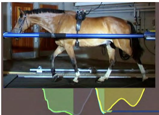
Abb. 3: Pferd im Schritt auf dem instrumentierten Laufband, das die Auffussungskräfte aller 4 Beine parallel misst. Kraftkurven unter dem Bild: Grün: Auffussungskräfte des linken Vorderbeins; Gelb: die Auffussungskräfte des rechten Hinterbeins. Die Vorderbeine tragen ca. 60% des Gewichtes, die Hinterbeine 40%.
